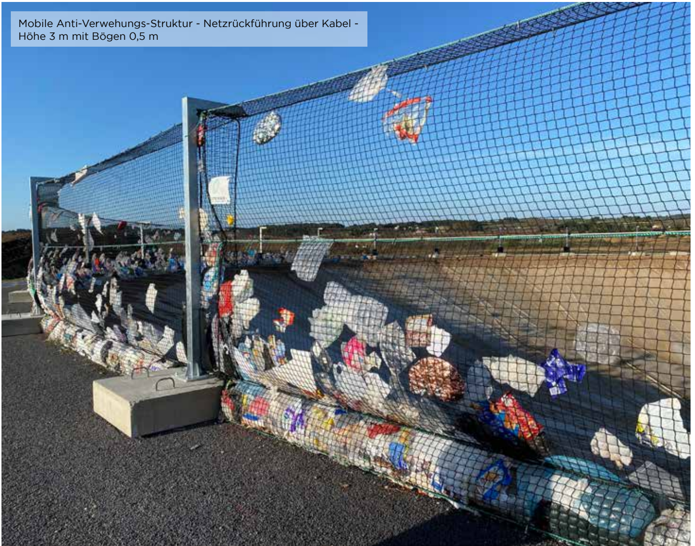
Mobiler Anti-Verwehungs-Käfig - große Dimensionen: Tiefe 60 m x Breite 40 m
